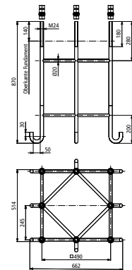
Maßbild
