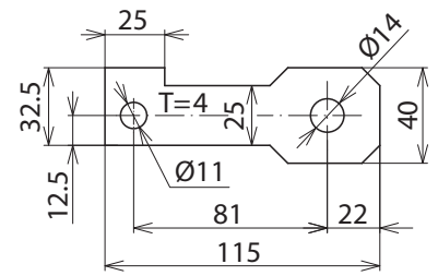
Maßbild AB EXFS IF3 G 14
