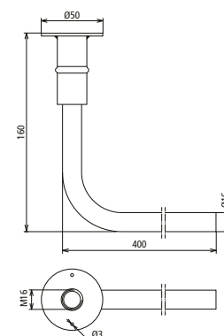
Maßbild D BEB 2 / EBS 15-03-19
