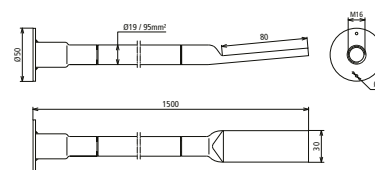
Maßbild D BEB 5 - L1500 / EBS 15-03-19
