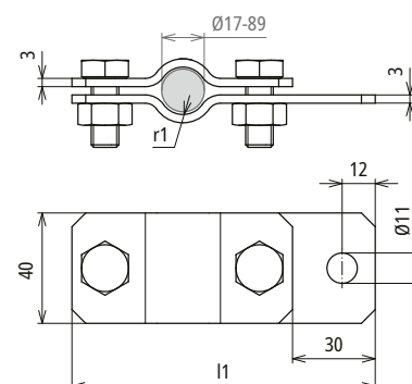
Maßbild ERS 48 AB11 STTZN
