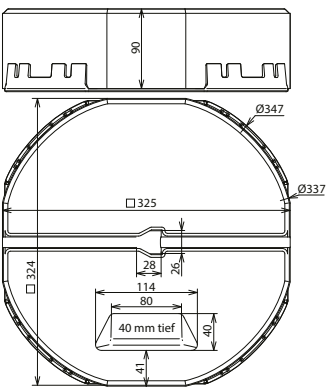
Maßbild BES 17KG KT16 ULP D337
