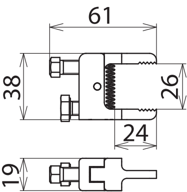
Maßbild KKS M8 0 24 SK10
