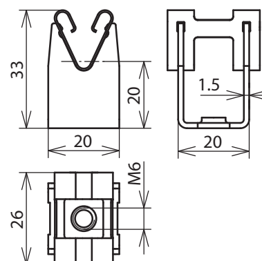
Maßbild LH DG 8 H20 IGM6 CU
