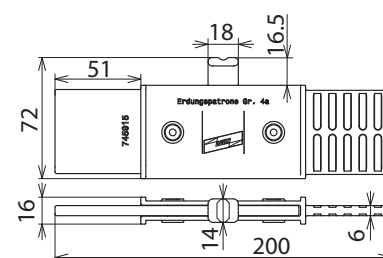
Maßbild EP NH4A VI TA
