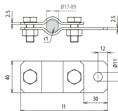
Maßbild ERS 55 AB11 V2A
