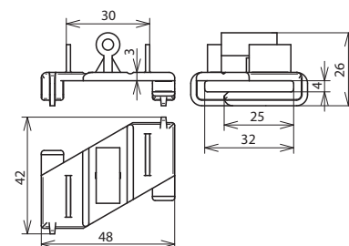
Maßbild FLA30 FB KF K SW
