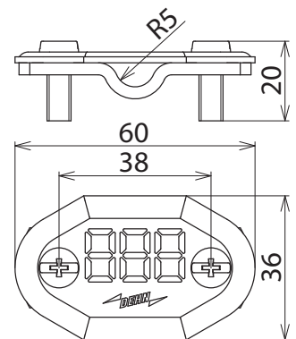
Maßbild NS 7.10 FL30 7SEG AL
