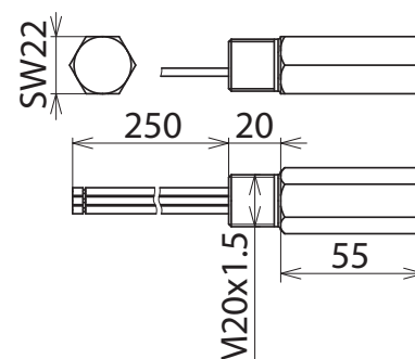
Maßbild DPI CD EXD 24 M
