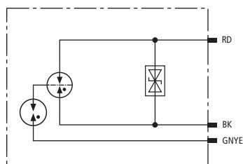
Prinzipschaltbild DPI CD EXD 24 M
