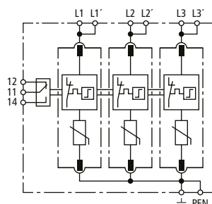
Prinzipschaltbild DG MP TNC 440 FM
