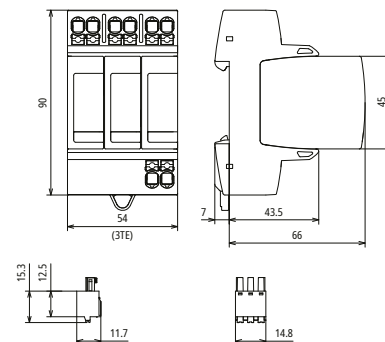
Maßbild DG MP TNC 440 FM
