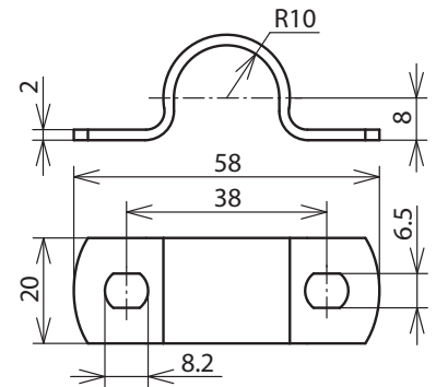
Maßbild LH ZSUEL 20 2XB6.5 V2A
