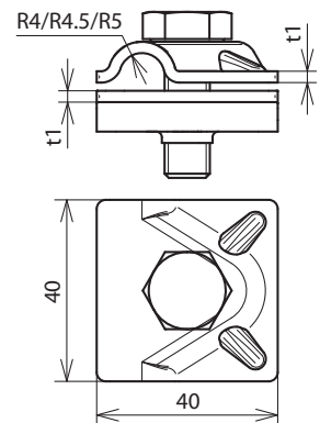
Maßbild MVK 10 SKM10X35 V4A
