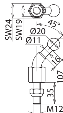
Maßbild KFP 20 W45 M12 35SSM
