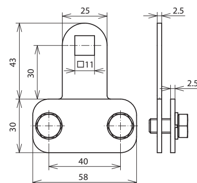
Maßbild KS 200 B11.11 FL30X4 V2A
