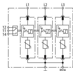
Prinzipschaltbild DG M TNC 440 FM
