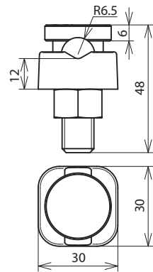
Maßbild KSV 8.12.5 STTZN
