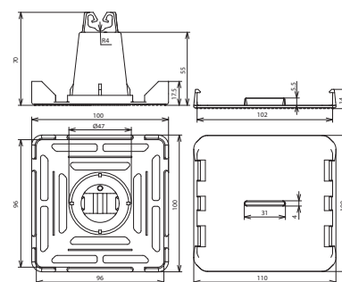
Maßbild DLH KF 8 LO DBS 110X100X70 SW
