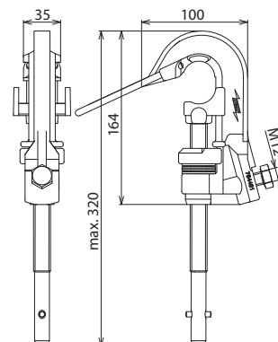
Maßbild PSK 4 30 SQL EH
