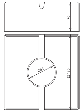
Maßbild BES 4.6KG SB10 180X180X70
