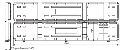
Maßbild KKL PHE3 60 110
