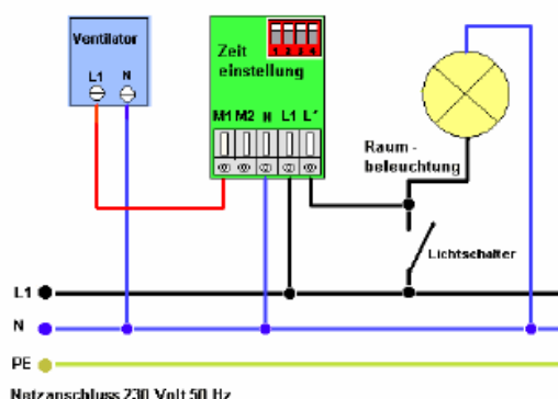
Einbau in Verteilerdose
