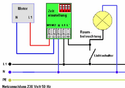
Einbau in Ventilator
