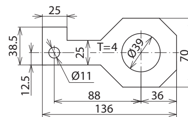
Maßbild AB EXFS IF3 G 39
