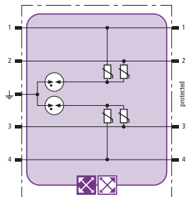
Prinzipschaltbild BXT ML4 MY 250
