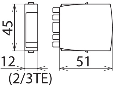
Maßbild BXT ML4 MY 250
