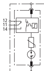
Prinzipschaltbild DG S 385 VA FM
