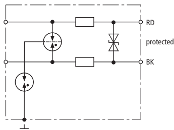
Prinzipialschaltbild DPI MD EX 24 M 2
