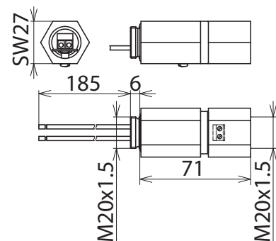
Maßbild DPI MD EX 24 M 2
