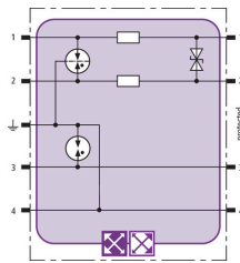
Prinzipialschaltbild BXT ML2 BD DL S 15
