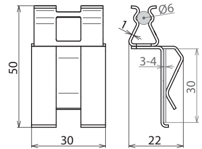
Maßbild DC BK 6 FL30 STBLANK
