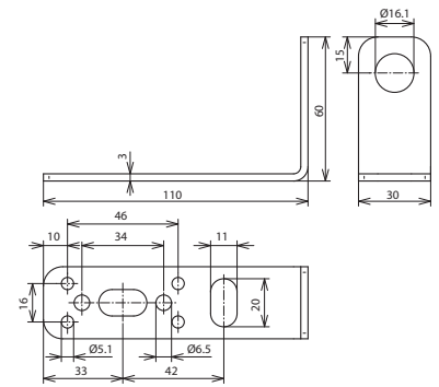
Maßbild BW90 B16 B5.1 6.5 11 V2A
