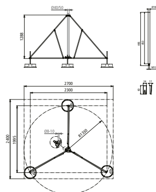
Maßbild DBS KB D50 RA1330 V2A
