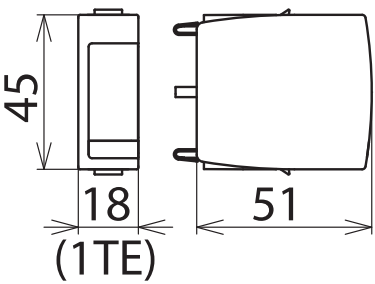
Maßbild DGP MOD DC Y 500
