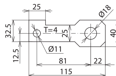
Maßbild AB EXFS IF3 G 18
