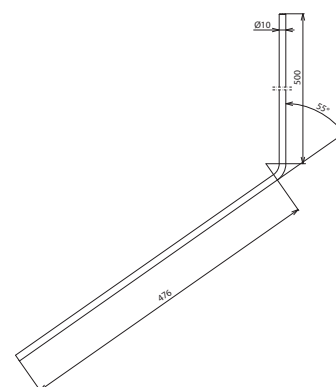
Maßbild FSP 10 1000 W55 AL
