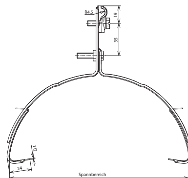
Maßbild DLH DQ 6.10 FG120.240 CU
