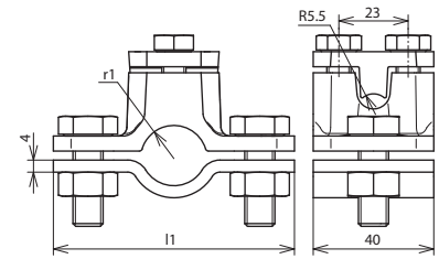
Maßbild ERS 48 AS4.10 TG STTZN
