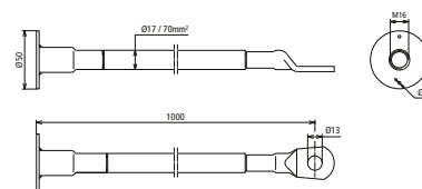
Maßbild D BEB 11 - L1000 / EBS 15-03-27
