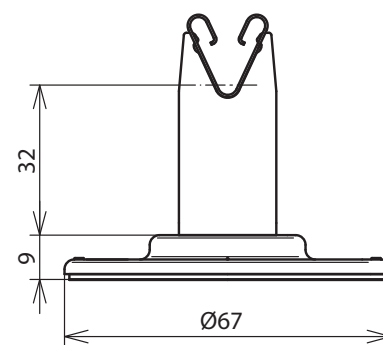
Maßbild DLH DG 8 H32 KP67 V2A K GR
