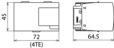
Maßbild DV MOD TT 255
