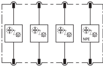
Prinzipschaltbild DV MOD TT 255
