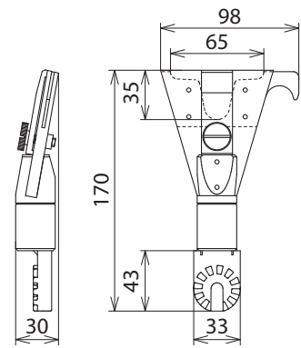
Maßbild AD ZK 3M 170
