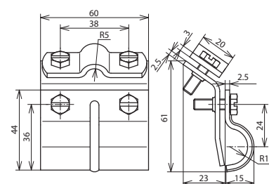
Maßbild DRK ZS 7.10 W13.25 B60 STTZN
