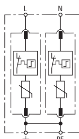
Prinzipschaltbild DG M TN 150
