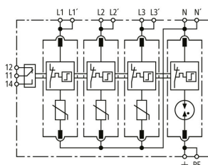
Prinzipialschaltbild DG MD TT 320 FM
