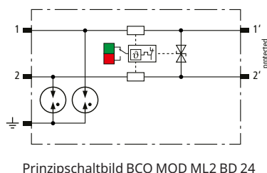
Prinzipschaltbild BCO MOD ML2 BD 24
