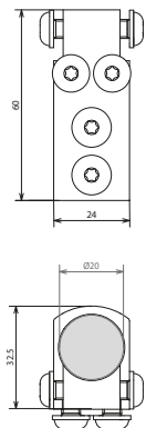
Maßbild AK TE 20 STGALZN
