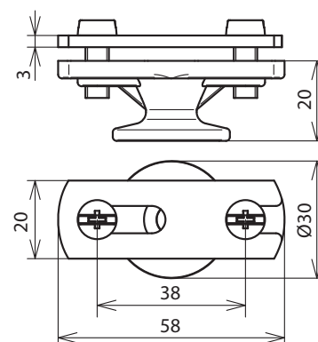
Maßbild FBH ZS 30 IGM8 STTZN ZG
