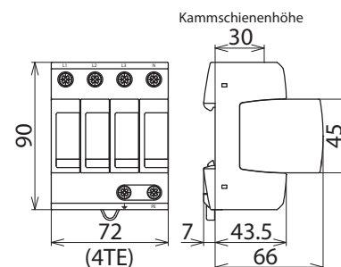
Maßbild DG M TNS 150
