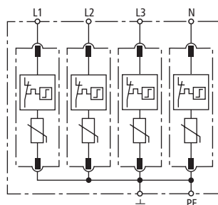
Prinzipschaltbild DG M TNS 150
