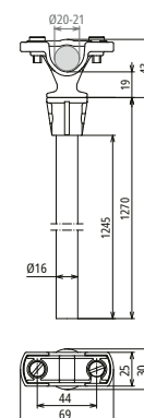
Maßbild DH ZS 20 D16 1270 GFK PA
